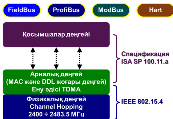
Сурет 2. Сымсыз автоматтандырудың деңгейлік құрылымы
