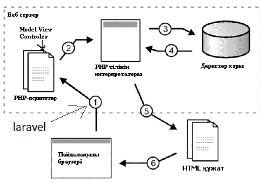
Сурет 1. Веб технология құралдарының өзара байланысы
