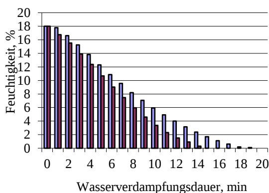
■ Feuchtigkeit der feinen Rohmischung, % ■ Feuchtigkeit der extrem groben Rohmischung, %
